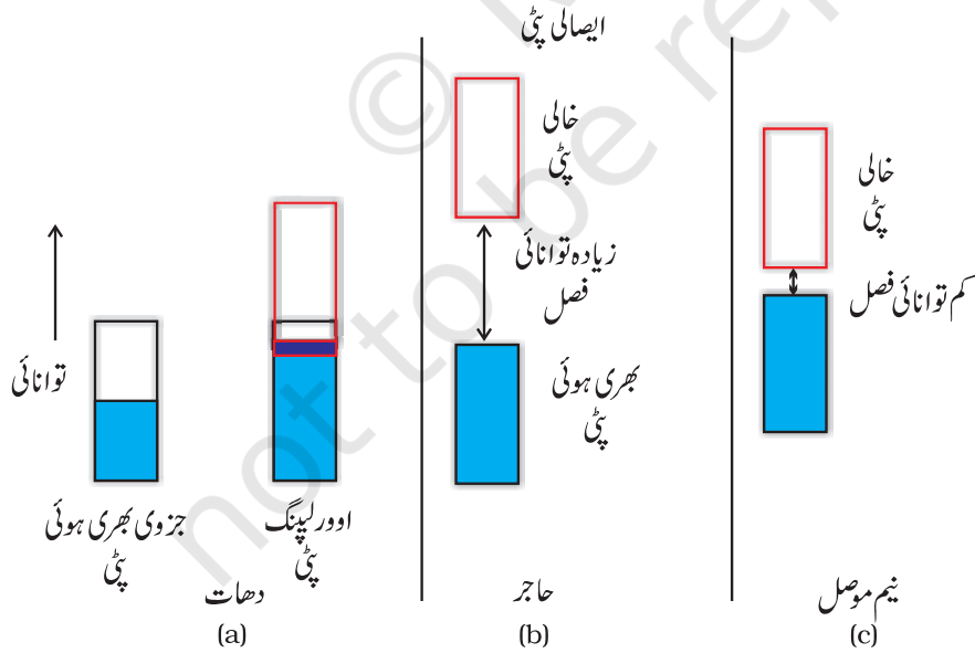
شکل 1.33 امتیاز مابین (a) دھات (b) عاجز اور (c) نیم موصل۔ ان میں سے ہر ایک صورت میں، بنا شیڈ کا حصہ ایصال پٹی کا اظہار ہے۔
