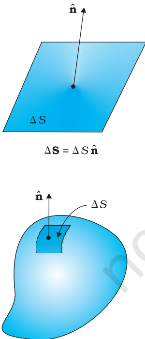
चित्र 1.19 अभिलंब \hat{\mathbf{n}} तथा \Delta S को परिभाषित करने की परिपाटी।
